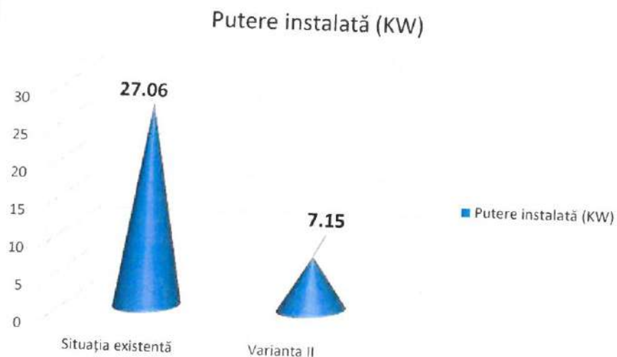
Fig. 14 Comparare putere totală instalată
