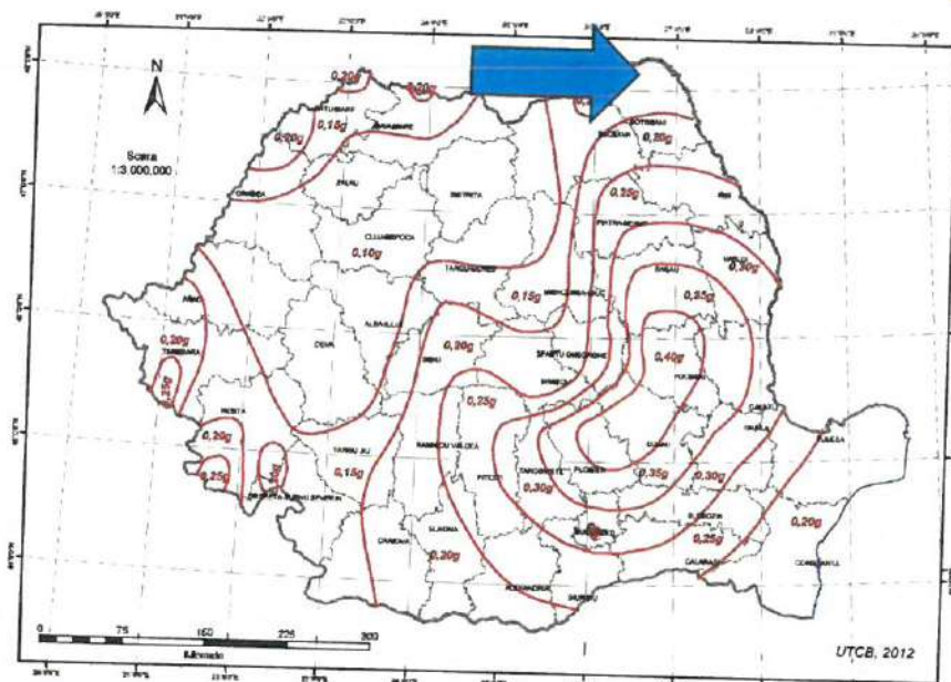
Fig. 6 – Zonarea accelerației terenului
