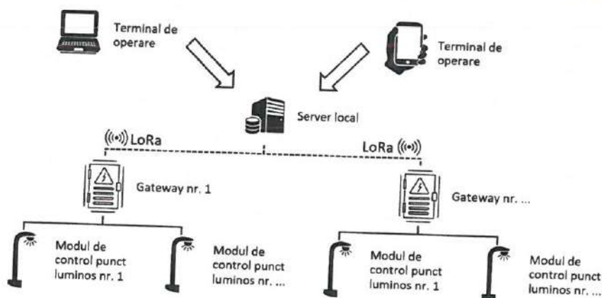
(Schema principiu de functionare)
