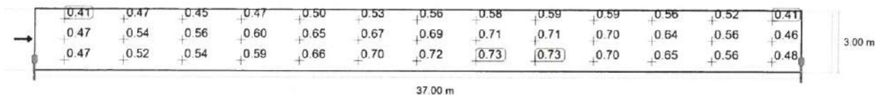
Observator 1: Valoarea de întreținere, densitatea luminii cu carosabil uscat [cd/m 2 ] (Raster valoric)
